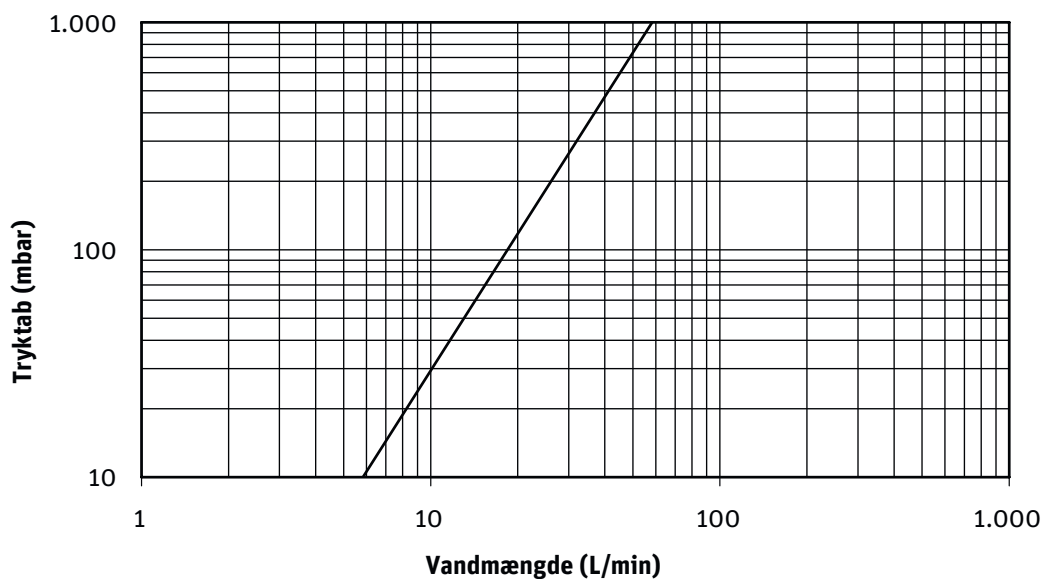
Tryktabsdiagram
